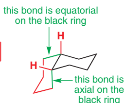
cis -decalin
